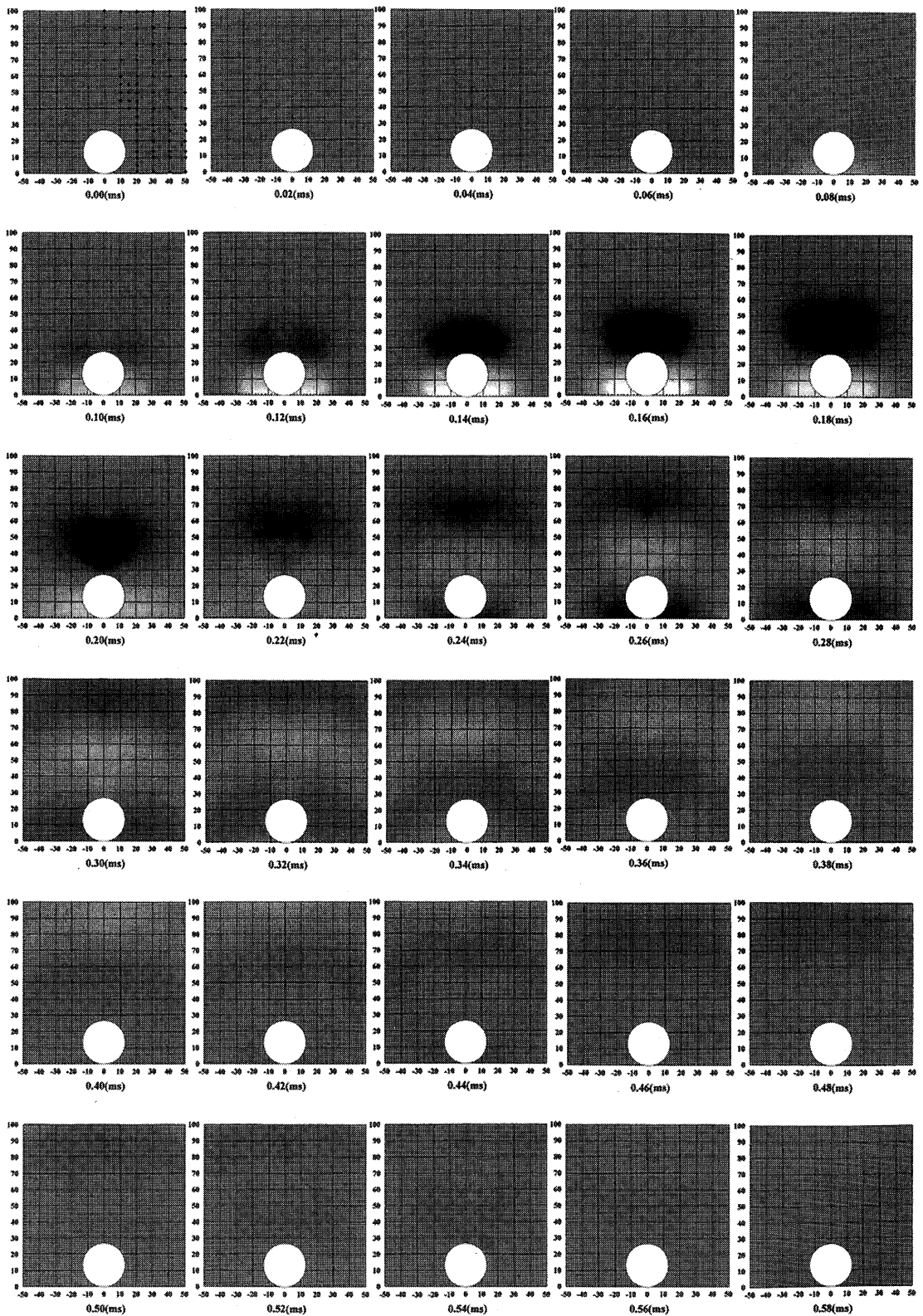
図-16 鋼球周辺の音場での音圧分布の連続図：M-5 供試体
