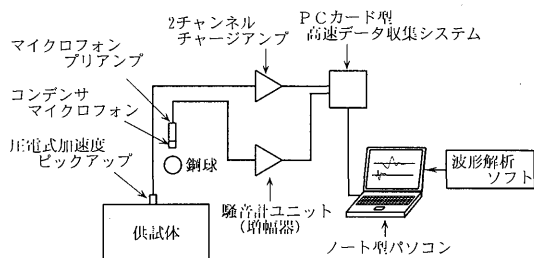
図-7 測定装置ブロックダイアグラム
