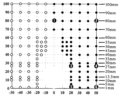
図-6(a) 測定したマイクロフォンの設置位置(黒塗り)
