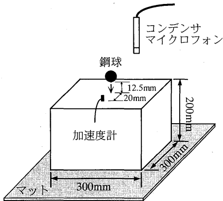
図-5 実験概念図
