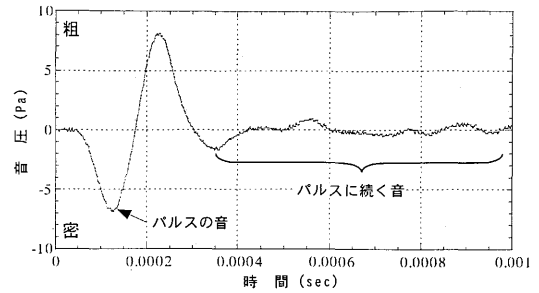
図-2 パルス音とパルスに続く音
