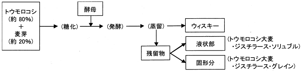
グレインウイスキーの製造工程 トウモロコシ大麦・ジステラース・グレインなどの生産フローシート
