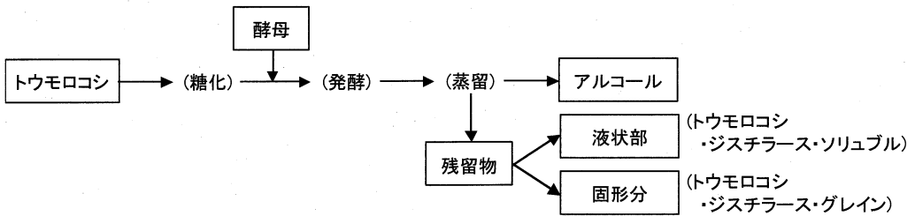
トウモロコシ・ジステラース・グレインなどの生産フローシート
