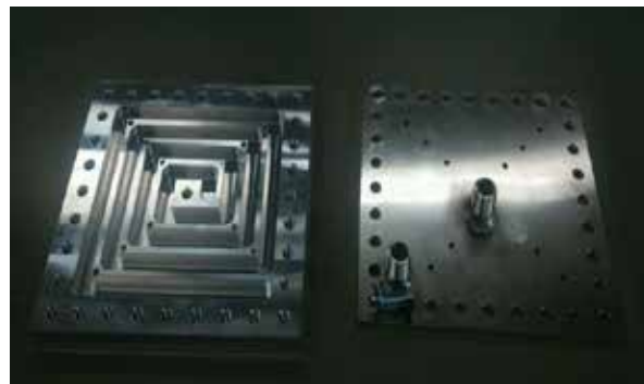
図4 完成した加熱部(左:受光面 右:底面)
