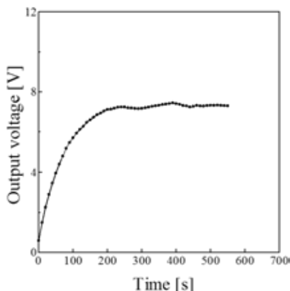
図 16 出力電圧 (L = 20 cm)
