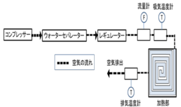
図5 装置構成図
