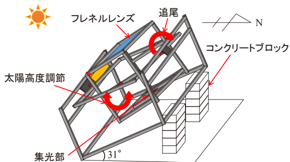
図1 フレネルレンズ式太陽集光装置の概略図
