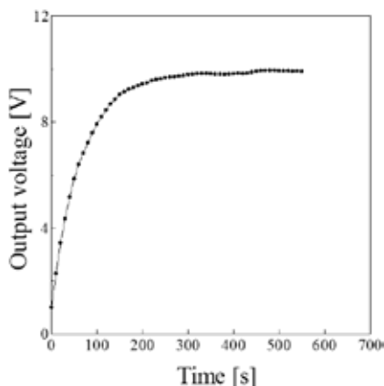
図 15 出力電圧 (L = 15 cm)
