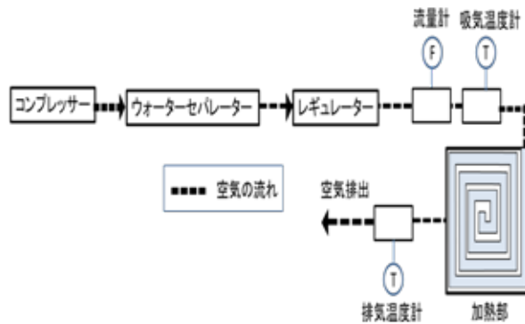
図5 装置構成図
