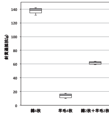
図6 実験用布の針貫通抵抗
