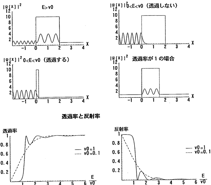
図2 凸型ポテンシャルでの散乱
