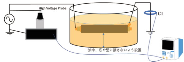
図2. 実験回路
