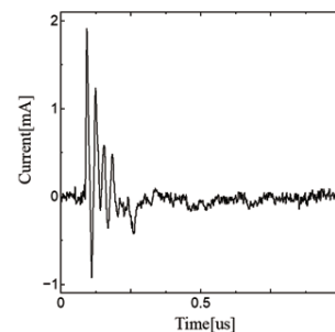
図 9 3 番ケーブル試験結果
