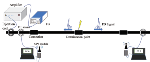
図1. 位置標定手法の概要
