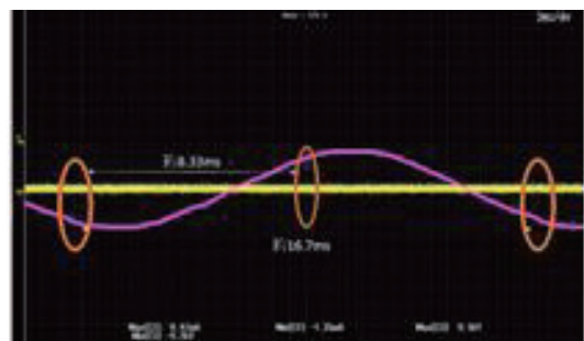
図4. 商用周波数と放電信号の関係
