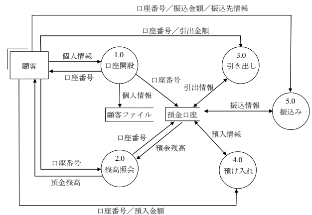
図 6 DFD の例
